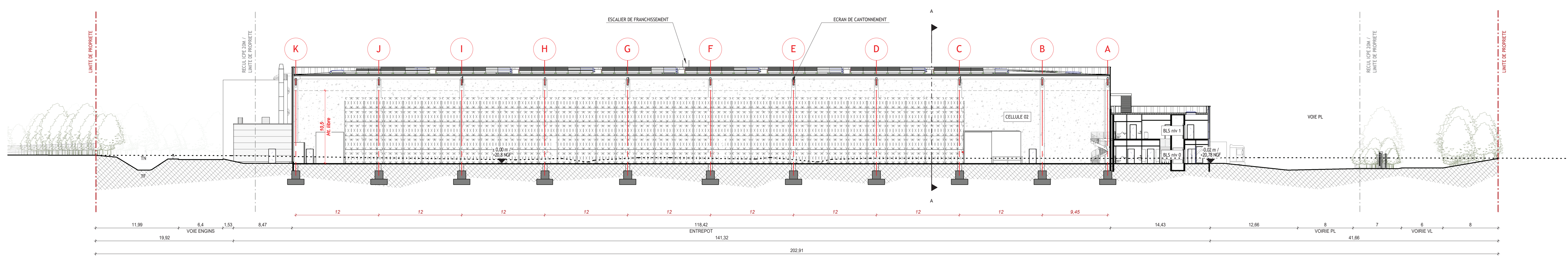
COUPE TRANSVERSALE BB Ech : 1 : 250
